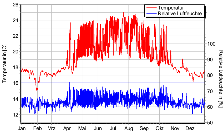
Temperatur- und Luftfeuchteverlauf für d_{Dä} = 30 mm, ohne Schlagregen (Nord) (Verlauf mit Schlagregen sehr ähnlich)
