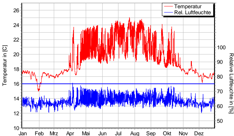
Temperatur- und Luftfeuchteverlauf für d_{D\ddot{a}} = 30 \text{ mm} und 1 SL, ohne Schlagregen (Nord) (Verlauf mit Schlagregen sehr ähnlich)
