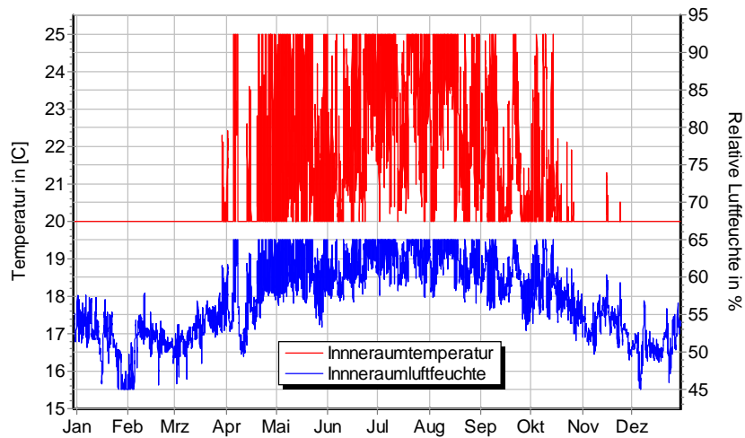
Abb. D.6: Raumklima: Stündliche Werte für Temperaturen (20-25°C) und relative Luftfeuchte (45-65%); entwickelt in Anlehnung an EN 15026 (s. Teil 1, 3.4.3)
