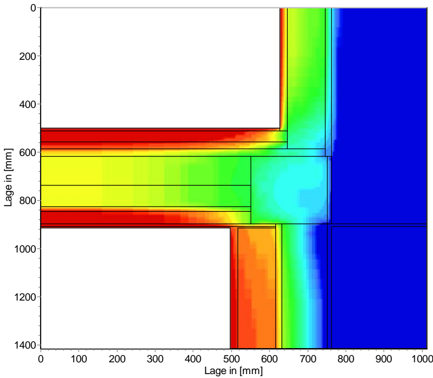
Relative Luftfeuchte - nass: Verteilung der Luftfeuchte am 23. März mit d_{D\ddot{a}} = 100 \text{ mm} , mit Schlagregen (West)
