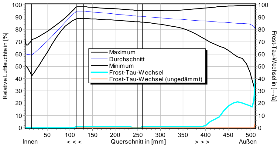
Luftfeuchteprofile und Frost-Tau-Wechsel für d_{D\ddot{a}} = 100 mm, ohne Schlagregen (Nord)
