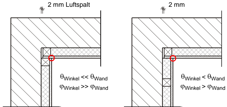
Abb. 0.2: Schnitt durch den Gebäudewinkel bei einem Dämmsystemen mit einer Holzträgerkonstruktion. Mit beiden Holzleisten im Winkel (links) hat die Dämmwirkung des eigentlichen Wärmedämmstoffs nur geringen Einfluss auf die Temperatur und Luftfeuchte im Gebäudewinkel, die Dämmwirkung der Holzleisten dominiert.
