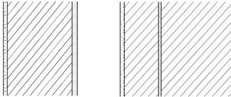
Abb. 0.1: Schematischer Aufbau der bestehenden, ungedämmten Grundkonstruktion: Links mit einer Steinlänge (1 SL) beidseitig verputzt, rechts mit 1½ Steinlängen (1½ SL) außenseitig unverputzt
