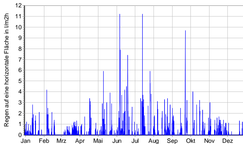
Abb. D.3: Stündliche Niederschlagsmengen auf eine horizontale Fläche: Jahresverlauf für Testreferenzregion 13 (Passau)
