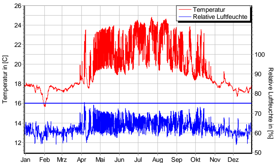
Temperatur- und Luftfeuchteverlauf für d_{D\ddot{a}} = 40 \text{ mm} , ohne Schlagregen (Nord) (Verlauf mit Schlagregen sehr ähnlich)
