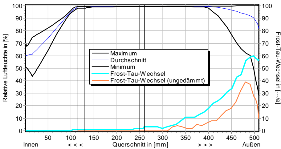
Luftfeuchteprofile und Frost-Tau-Wechsel für d_{D\ddot{a}} = 100 mm, schlagregenexponiert (West)
