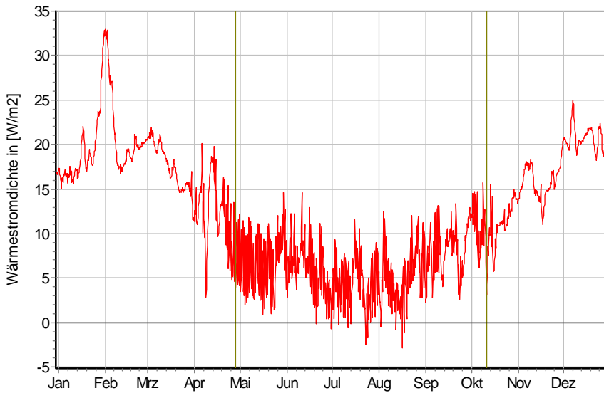
Wärmestromdichte über Innenwandoberfläche für d_{D\ddot{a}} = 40 \text{ mm} , ohne Schlagregen (Nord) Heizperiode vom 8. Oktober bis 29. April (Verlauf mit Schlagregen sehr ähnlich)
