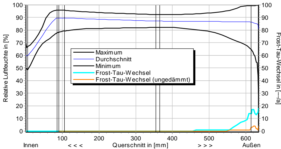
Luftfeuchteprofile und Frost-Tau-Wechsel für d_{D\ddot{a}} = 80 \text{ mm} , ohne Schlagregen (Nord)
