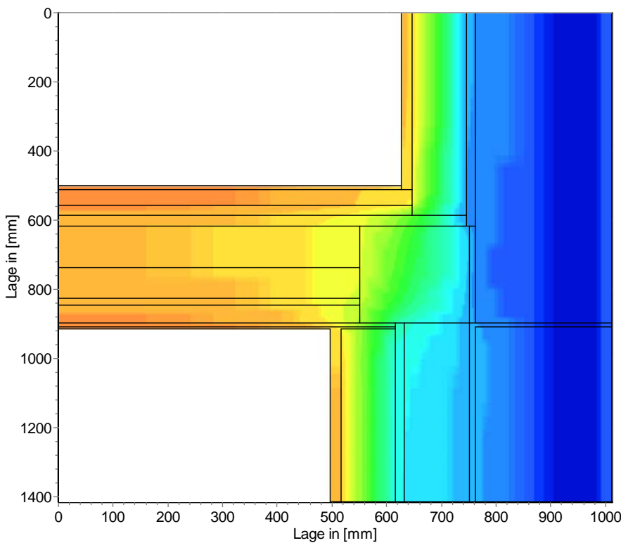
Temperatur - kalt: Temperaturverteilung am 2. Februar mit d_{D\ddot{a}} = 100 \text{ mm} , ohne Schlagregen (Nord)
