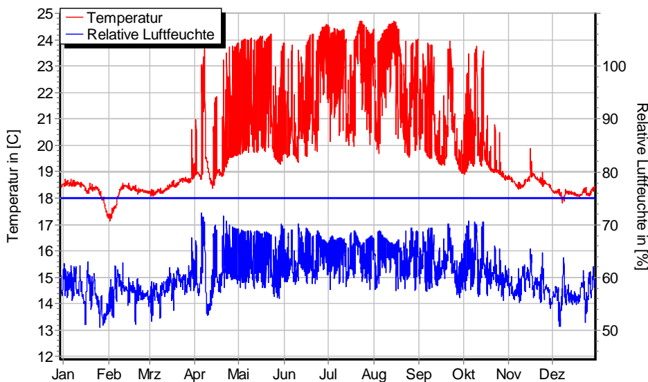
Temperatur- und Luftfeuchteverlauf für d_{D\ddot{a}} = 30 \text{ mm} , ohne Schlagregen (Nord) (Verlauf mit Schlagregen sehr ähnlich)
