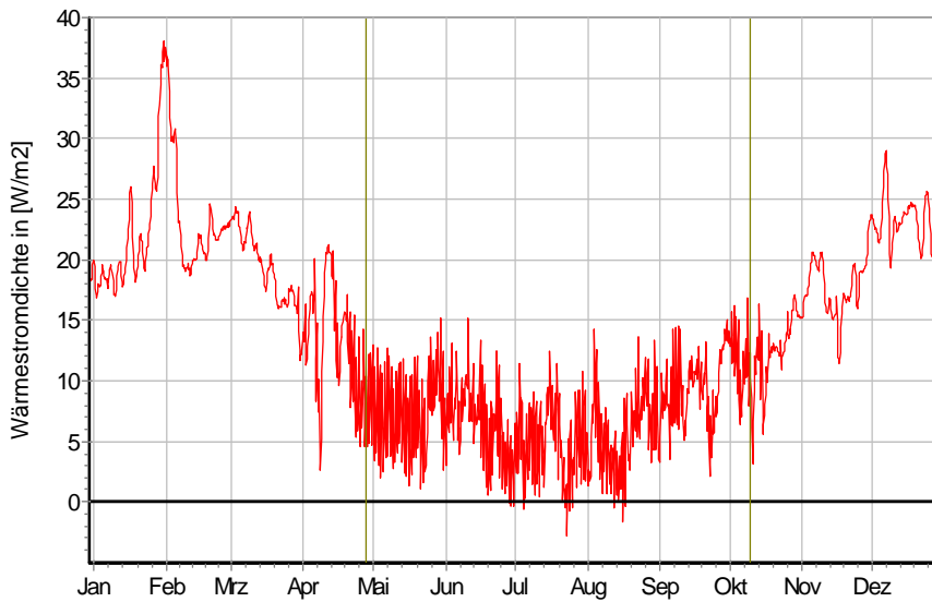
Wärmestromdichte über Innenwandoberfläche für d_{D\ddot{a}} = 30 \text{ mm} , ohne Schlagregen (Nord) Heizperiode vom 8. Oktober bis 29. April (Verlauf mit Schlagregen sehr ähnlich)
