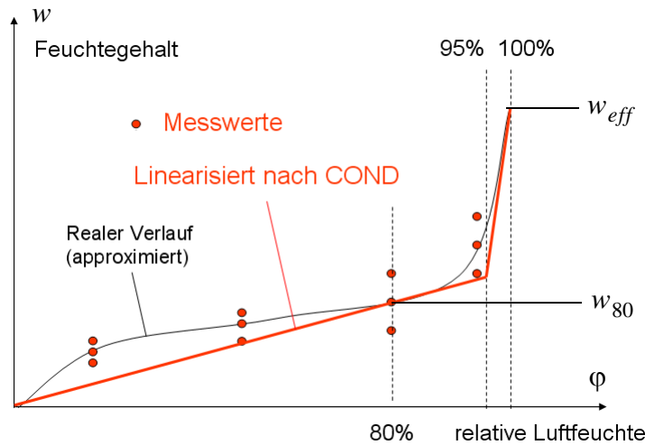
Abb. 2.3: Linearisierte Sorptionsisotherme
