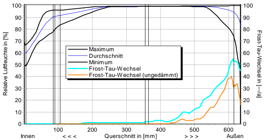
Luftfeuchteprofile und Frost-Tau-Wechsel für d_{D\ddot{a}} = 80 \text{ mm} , schlagregenexponiert (West)
