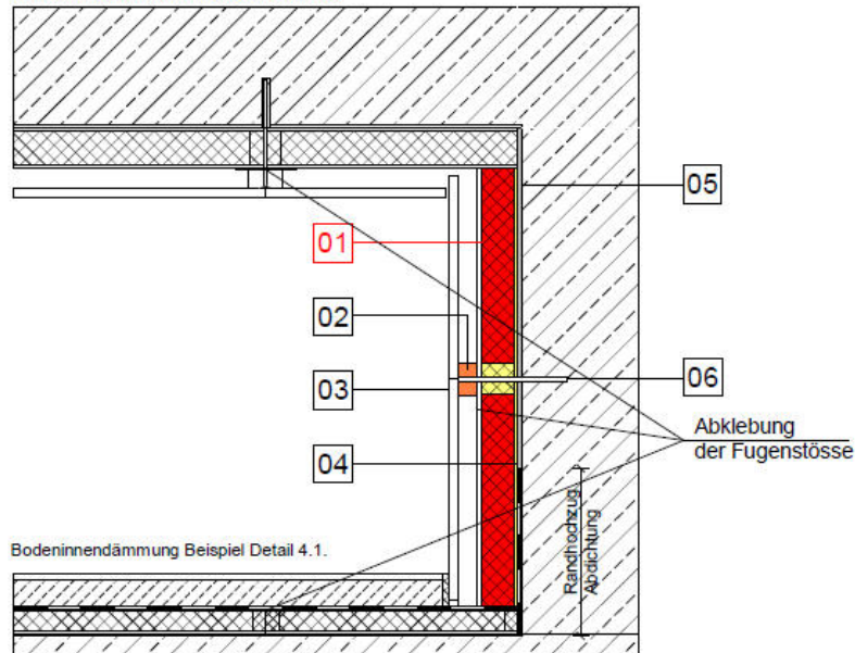
Deckeninnendämmung: Beispiel Detail 4.8.
